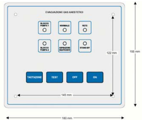
FJERNBETJENINGSPANEL, FOR NEM VAKUUMKONTROL OVER LANGE AFSTANDE FRA CENTRALEN. FJERNBETJENINGS DIMENSIONER: 180 X 155MM
